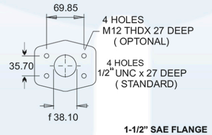
1-1/2" SAE FLANGE
