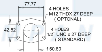
2" SAE FLANGE
